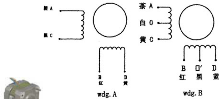
接线图(WIRING DIAGRAM)
